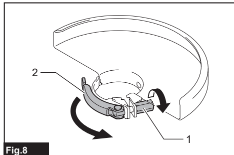
► 1. Nut 2. Lever
